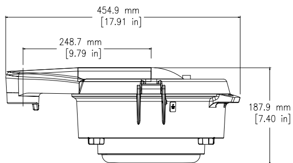
Vue latérale - Globe
