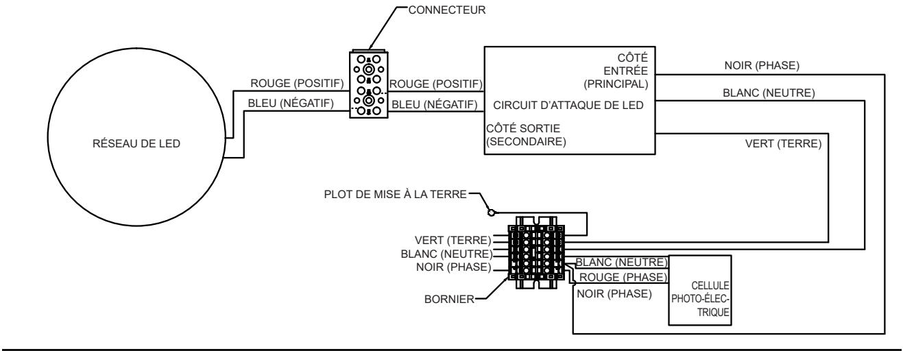
FIGURE 22 : LUMINAIRE AVEC INTERRUPTEUR PHOTOÉLECTRIQUE EN OPTION
