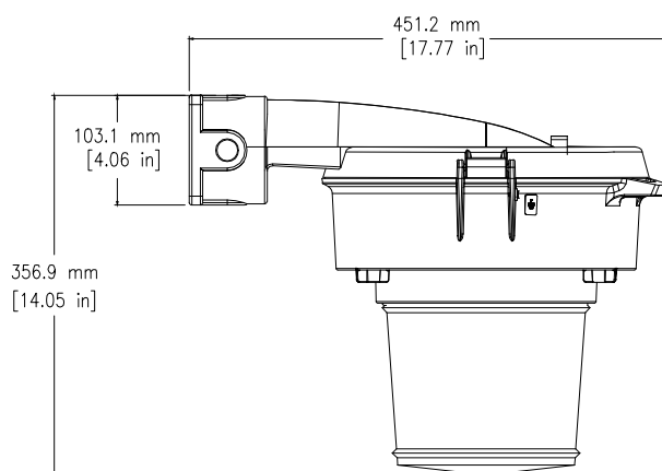
Vue latérale - Réfracteur (LPGR5)
