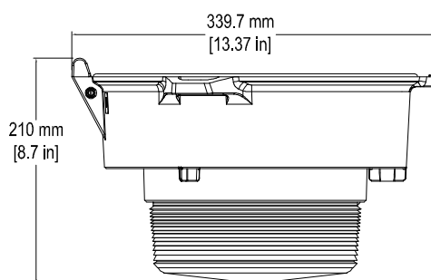
Vue latérale - Refracteur (LPGR5S)
