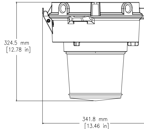
Vue latérale - Réfracteur (LPGR5)
