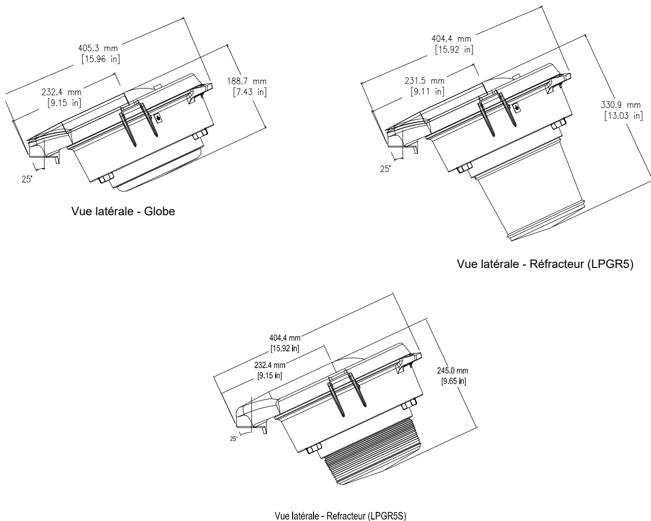
FIGURE 15 : LUMINAIRE AVEC CAPOT À COLONNE INCLINÉE À 25°
