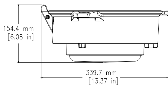
Vue latérale -Globe
