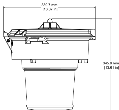
Vue latérale - Réfracteur (LPGR5)
