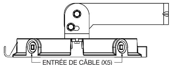
FIGURE 12 : DÉTAILS DU CAPOT À TOURILLON
