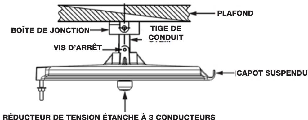
FIGURE 5 : DÉTAILS DU CAPOT SUSPENDU (VERSION ÉTANCHE À 3 CONDUCTEURS)
