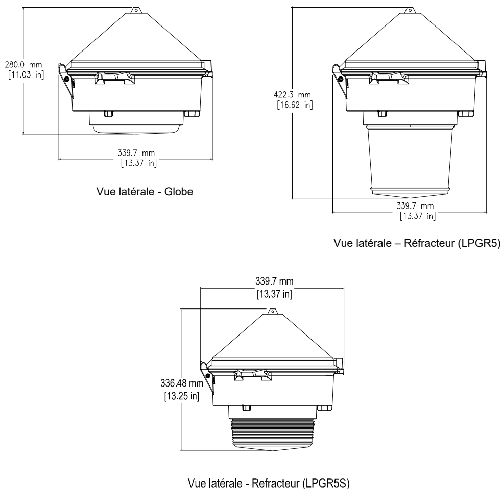
FIGURE 7 : LUMINAIRE AVEC CÔNE SUSPENDU
