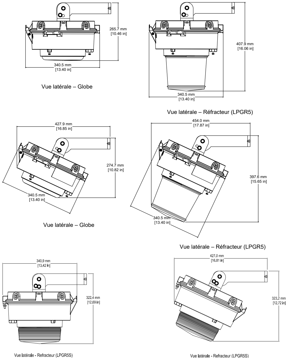
FIGURE 11 : LUMINAIRE AVEC CAPOT À TOURILLON
