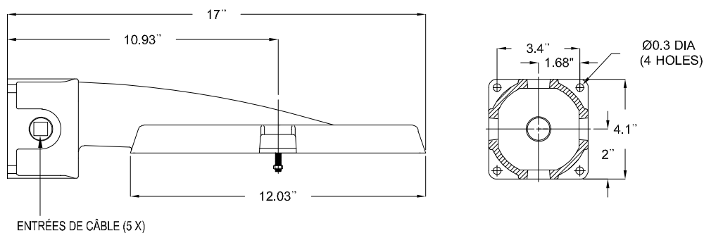
FIGURE 14 : DÉTAILS DU CAPOT MURAL
