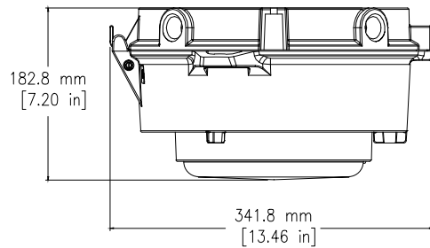
Vue latérale - Globe
