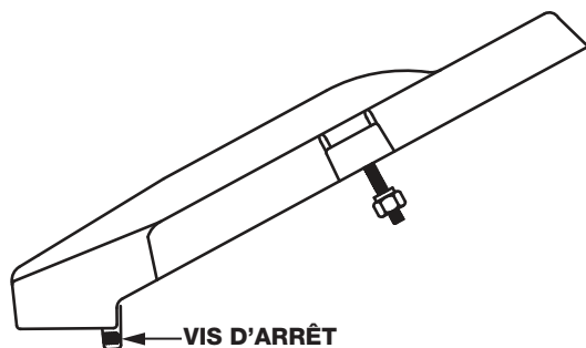
FIGURE 16 : DÉTAILS DU CAPOT À COLONNE INCLINÉE À 25°
