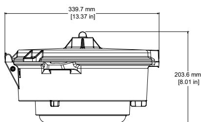
Vue latérale - Globe
