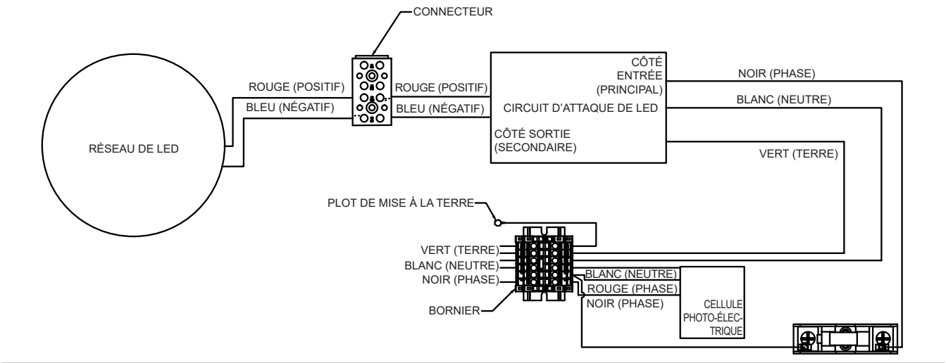
FIGURE 23 : LUMINAIRE AVEC INTERRUPTEUR PHOTOÉLECTRIQUE ET FUSIBLE EN OPTION
