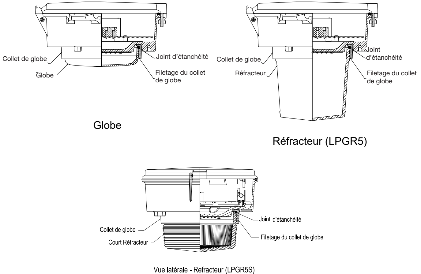
FIGURE 24 : DÉTAIL DE L'ÉTANCHÉITÉ DU GLOBE/RÉFRACTEUR
