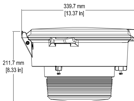
Vue latérale - Refracteur (LPGR5S)
