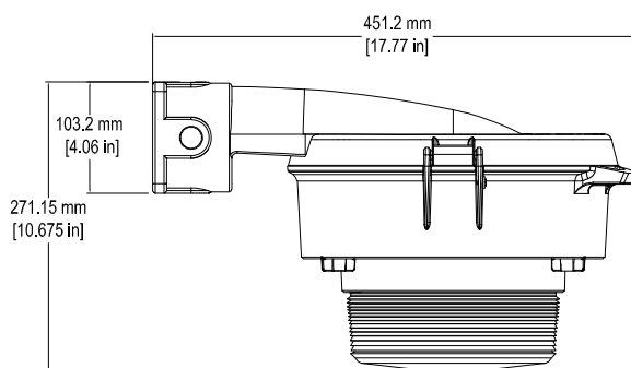
Vue latérale - Refracteur (LPGR5S)
