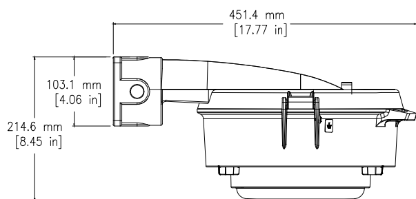
Vue latérale - Globe
