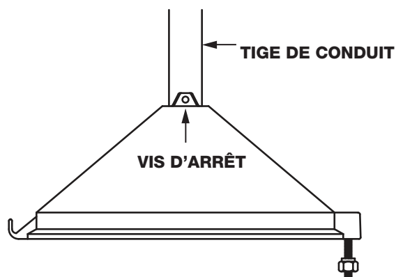
FIGURE 8 : DÉTAILS DU CAPOT À CÔNE SUSPENDU
