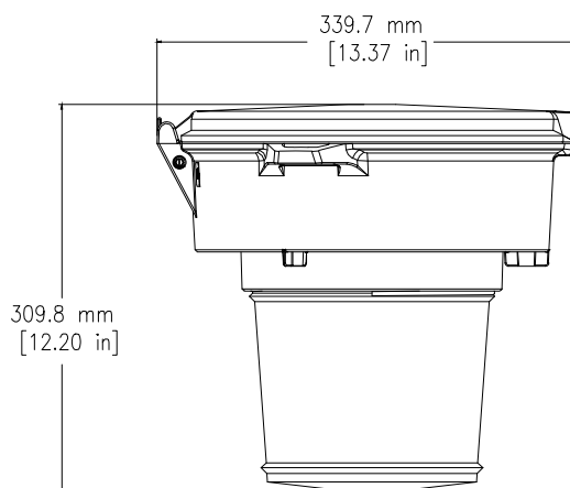
Vue latérale- Réfracteur (LPGR5)
