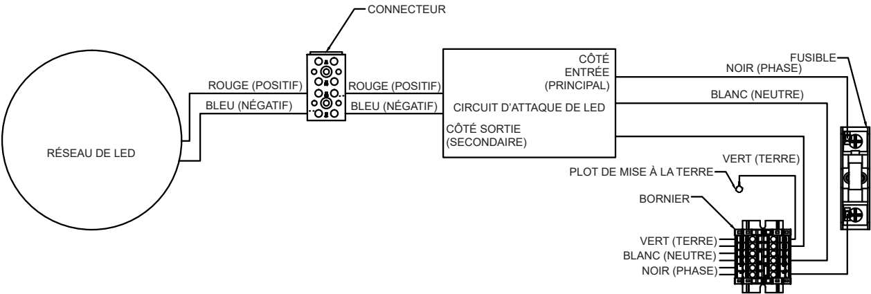
FIGURE 20 : LUMINAIRE
