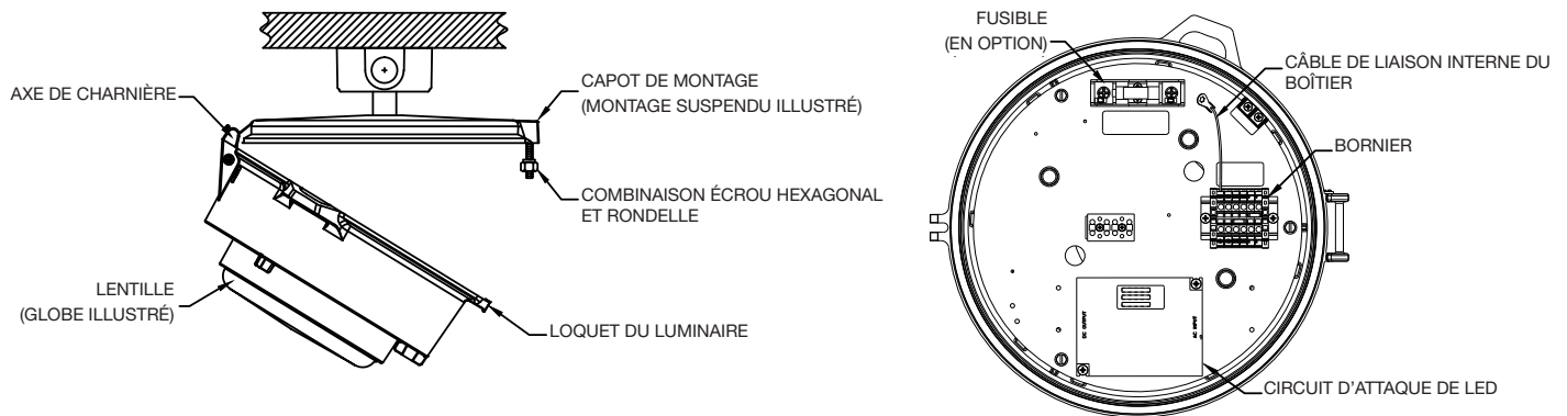
FIGURE 19 : COMPARTIMENT DE CÂBLAGE
