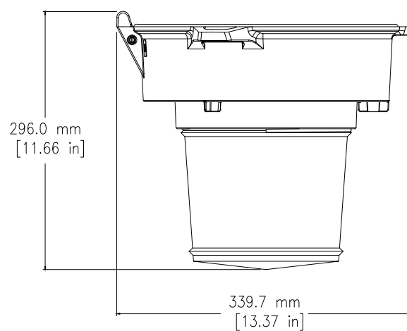
Vue latérale – Réfracteur (LPGR5)
