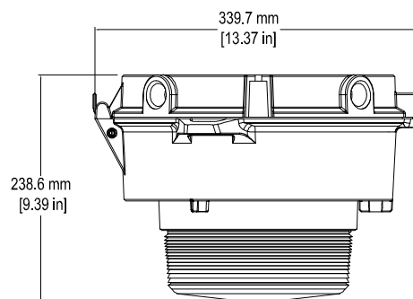
Vue latérale - Réfracteur (LPGR5S)
