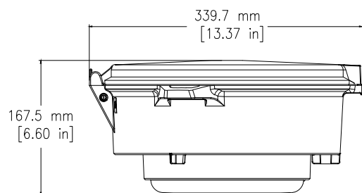
Vue latérale – Globe
