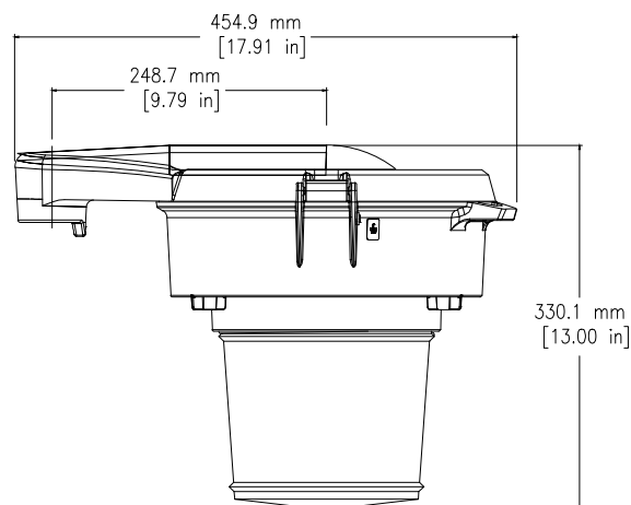
Vue latérale - Réfracteur (LPGR5)
