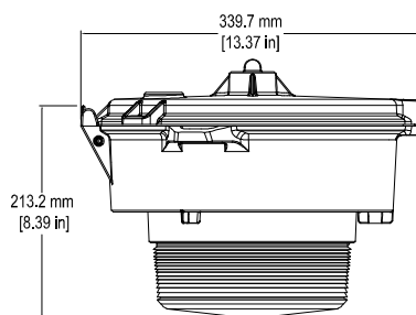
Vue latérale - Réfracteur (LPGR5S)
