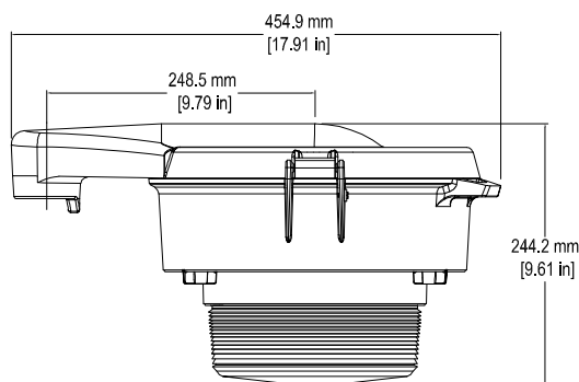
Vue latérale - Réfracteur (LPGR5S)
