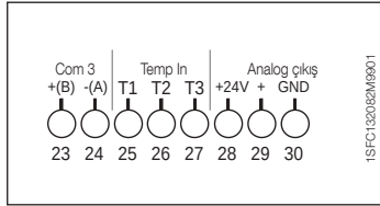
Şekil 2: Terminal bağlantısı
