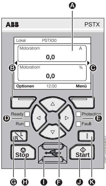
Abbildung 3: Display
