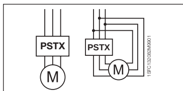
Kuva 1: Suorakytkentä, kolmiokytkentä
