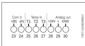
Obrázek 2: Připojení svorek
