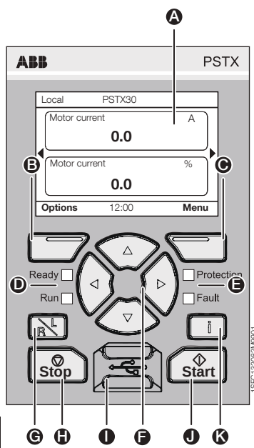
Afbeelding 3: HMI
