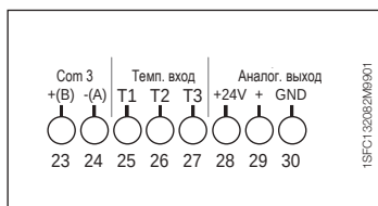
Рис. 2. Подключение контактов
