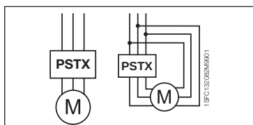
Рис. 1. Включение «в линию», включение в соединение «треугольником»
