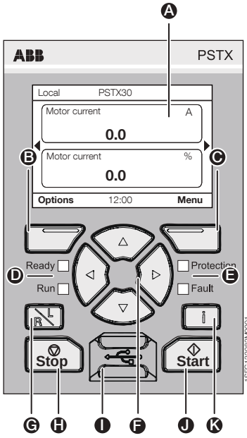
Şekil 3: HMI
