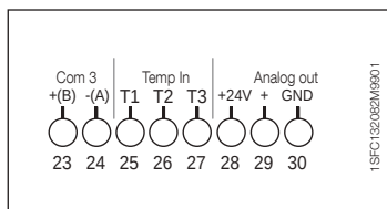
Afbeelding 2: Aansluiting aansluitklemmen
