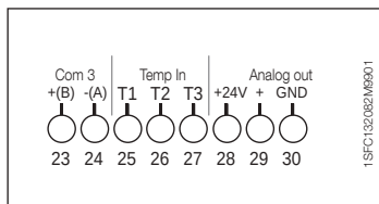
Kuva 2: Liittimen liitännät
