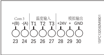
图 2：端子连接
