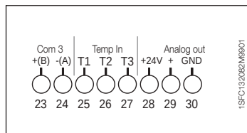
Abbildung 2: Klemmenanschluss
