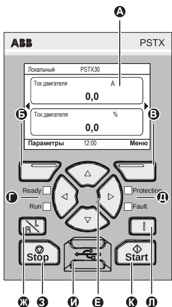
Рис. 3. Панель управления
