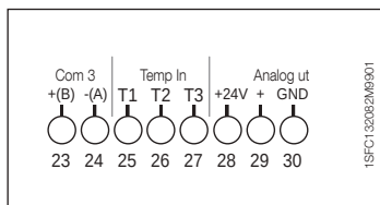
Bild 2: Plintanslutning
