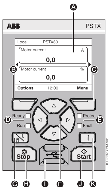
Obrázek 3: HMI
