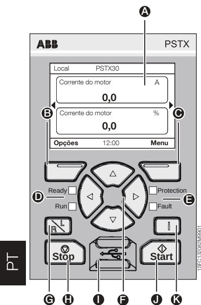
Figura 3: IHM
